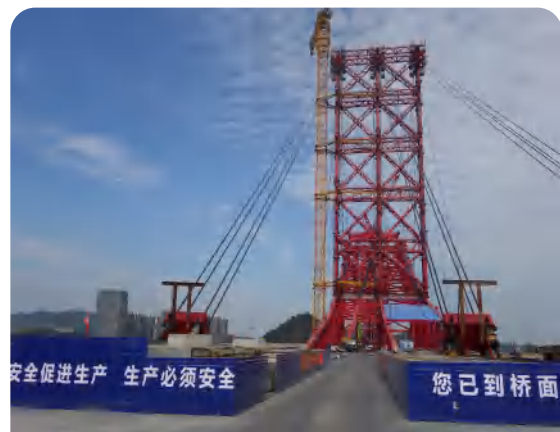
桥面作业区
