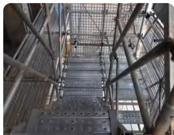
盘扣脚手架上下通道
