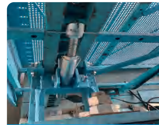
爬架防坠装置
