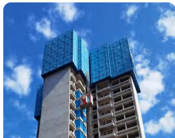
爬架外观
