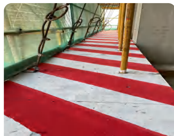
悬挑层封闭
