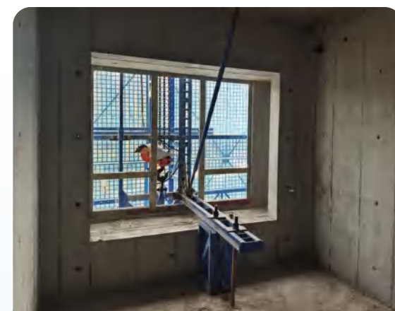
爬架板式支座
