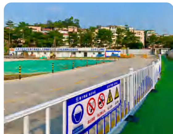
人车分流
